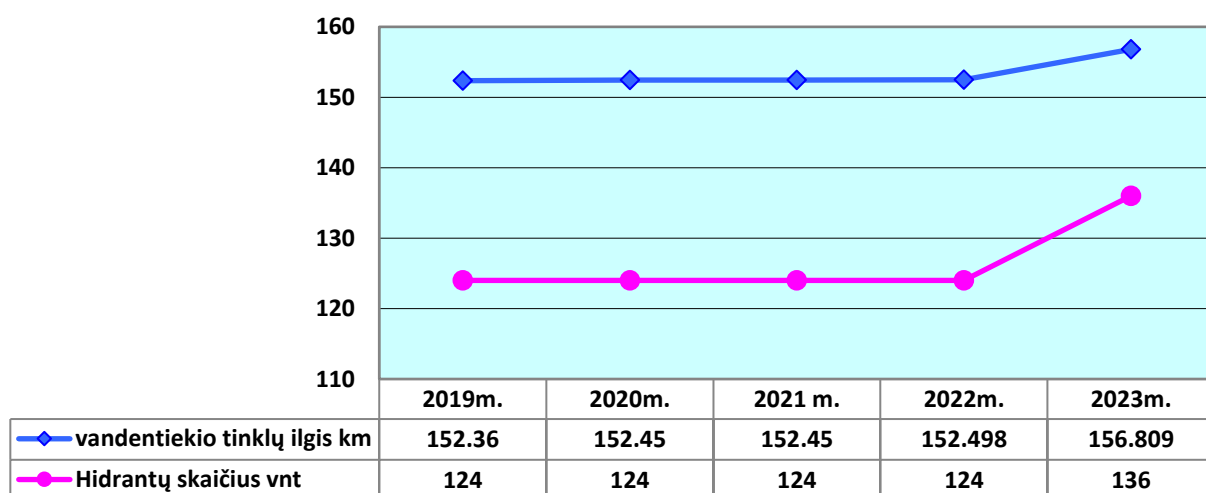
5 pav. Eksploatuojami vandentiekio tinklai ir hidrantai
